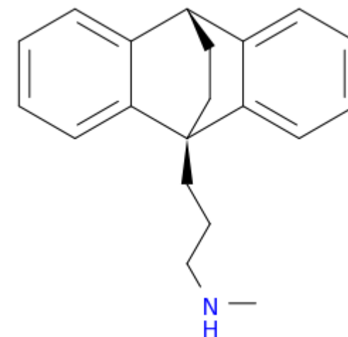
Maprotiline
