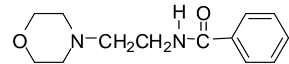
Moclobemide
