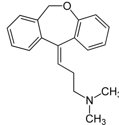
Cis Doxepin
