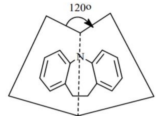
Dibenzazepine (Antidepressant)
