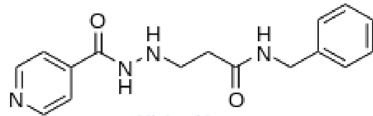
Nialamide
