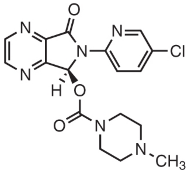
Eszopiclone
