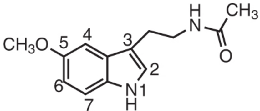
Melatonin
