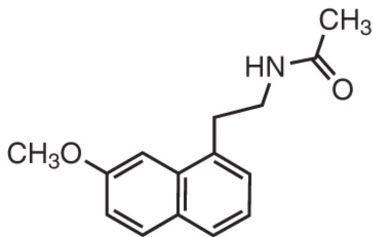
Agomelatine
