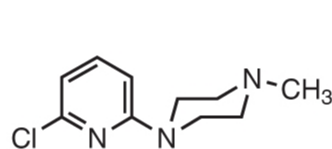
N-Me 6CPP
