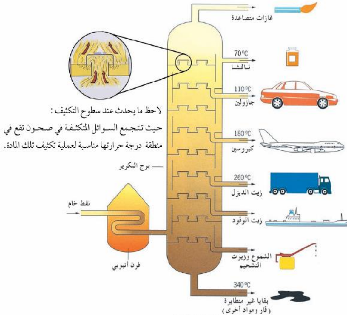
شكل (١٣-١٣): النواتج الأساسية لعمليات تقطير النفط
