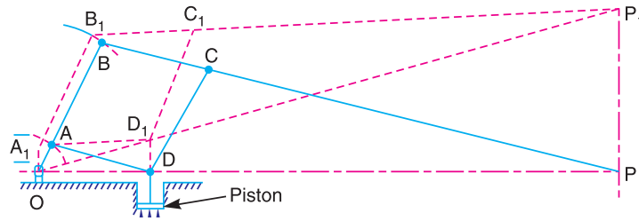
Fig. 9.11. Simplex indicator.
