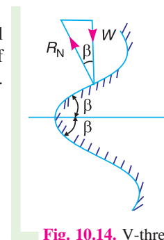
Fig. 10.14. V-thread.
