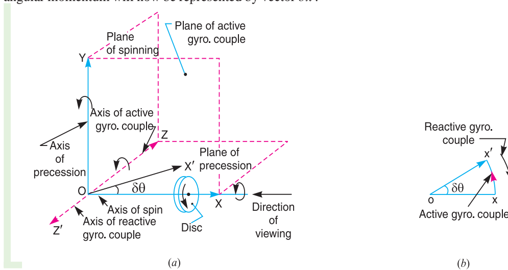
Fig. 14.2. Gyroscopic couple.
